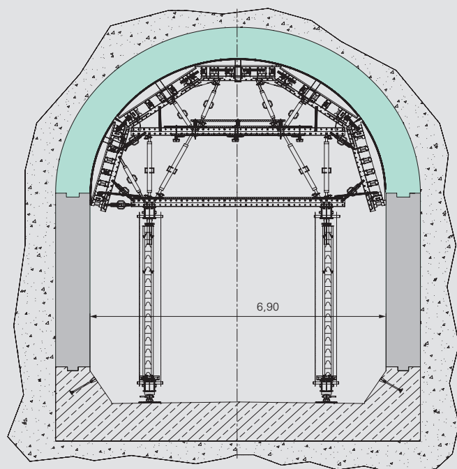
Również przejezdne deskowanie trzeciego etapu (odcinek sklepienia) odpowiada wymogom budowy.
